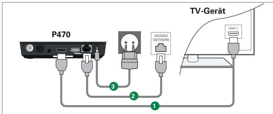
Abbildung 2 - Kabelverbindungen
